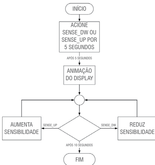
Figura 4 – Árvore de programação do Sense Funcionamento
