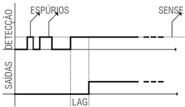
Figura 7 – Funcionamento do parâmetro Lag
