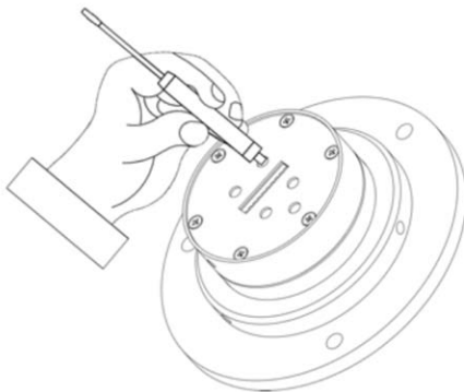
Figura 3 – Acionando um sensor magnético
