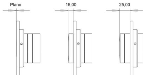
Figura 17 Configurações do flange
