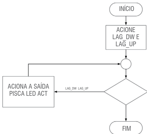
Figura 15 Acionando o Loop-test
