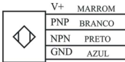
Figura 14 – Diagrama de conexão
