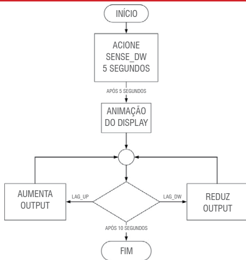
Figura 11 Árvore de programação do Output
