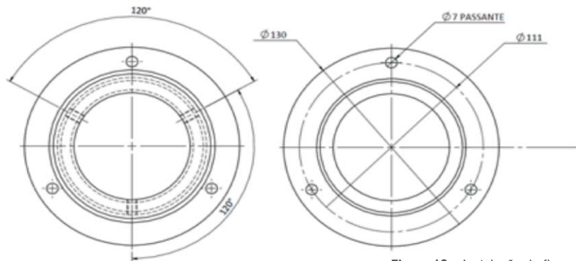
Figura 16 – Instalação do flange
