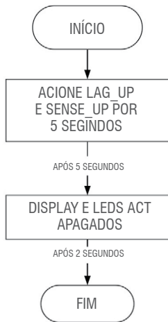
Figura 12 – Árvore de programação para reiniciar o SLV-1A
