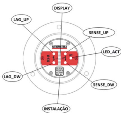
Figura 2 – Itens da interface
